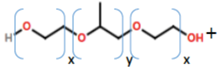
Poloxamer 407
